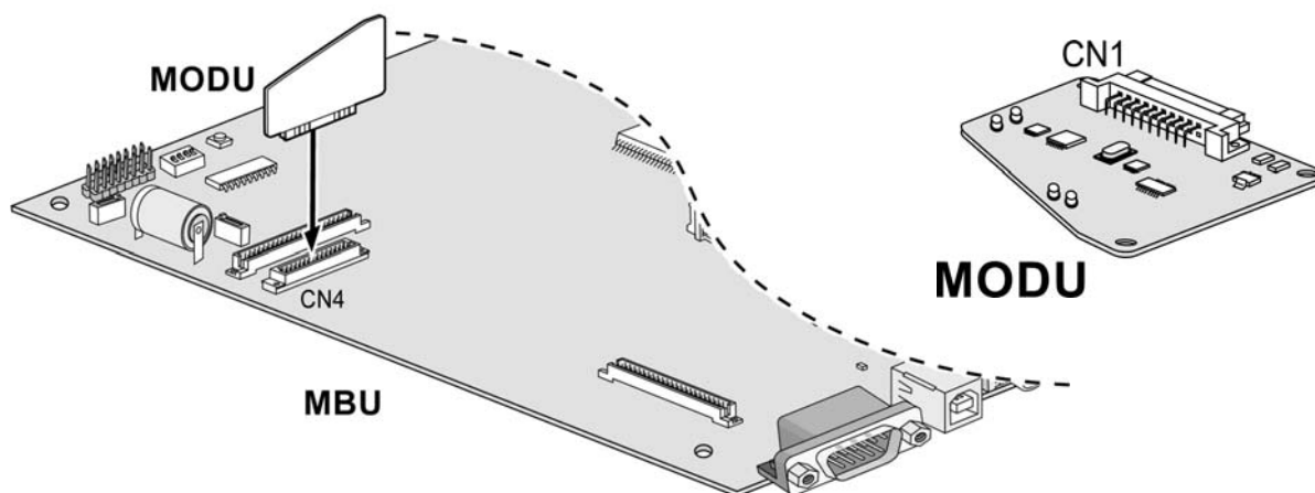
Рис. 2.18 Модуль внутреннего модема MODU
