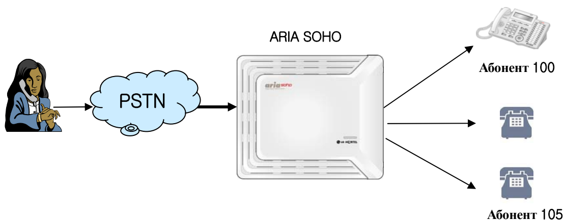
Рис. 3.2 Назначение приема входящих вызовов
