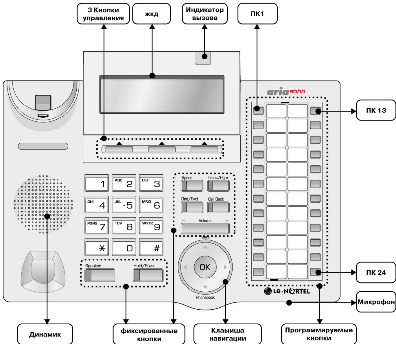
Рис. 3.1 Описание клавиш цифрового аппарата LDP-7224D
