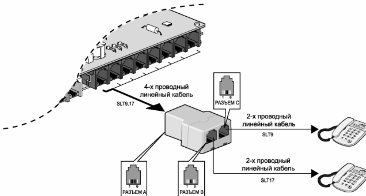
Рис. 4.4.2.2 Терминальный переходник
