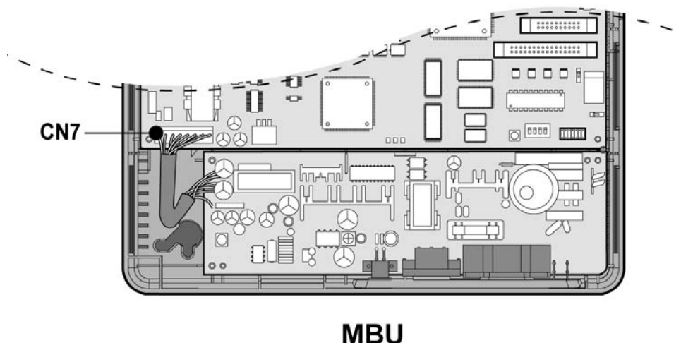
Рис. 3.2.4а Установка блока питания
