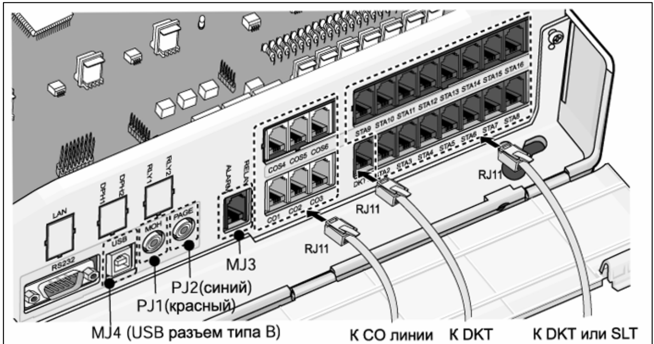
Рис. 4.26 Подключение
