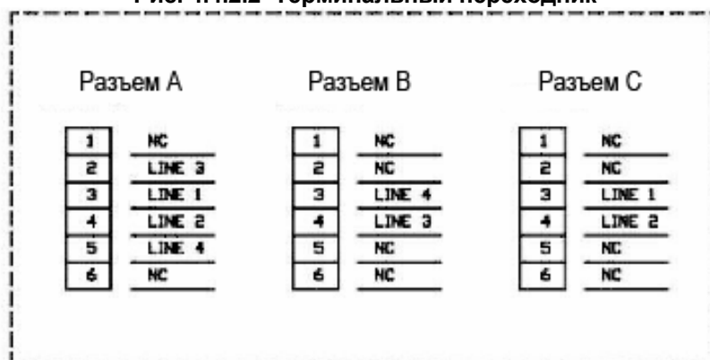
Рис. 4.4.2.2 Терминальный переходник
